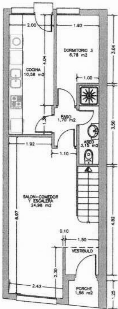
PLANTA BAJA
