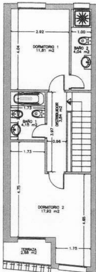
PLANTA ALTA
