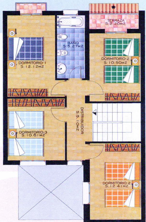
PLANTA PRIMERA
